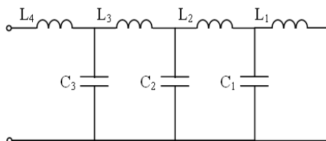
Рис. 4. Схема реактивного двополюсника, що відповідає динамічній механічній системі з чотирма масами
