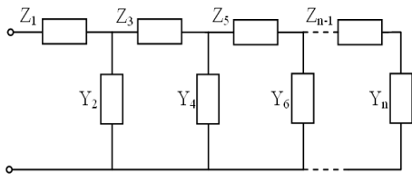
Рис. 3. Схема реактивного двополюсника
