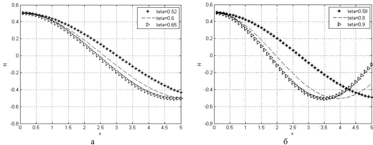
Рис. 1. Профіли свободної поверхні H(x) для величини відхилення емкості від початкового положення: а – \theta = 0.52; 0.6; 0.65 ; б – \theta = 0.58; 0.8; 0.9
