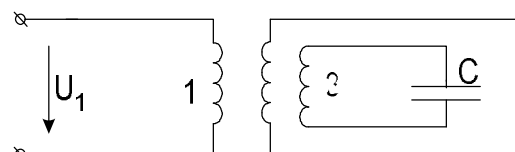
Рис. 2. Схема заміщення АГ
