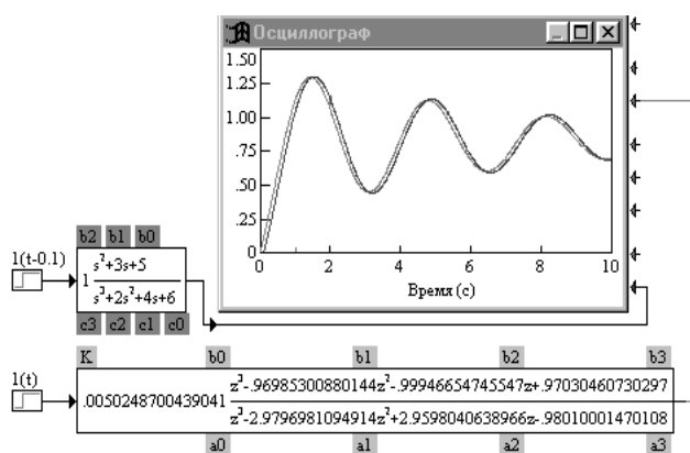
Рис. 2. Модель КІХ-фільтра у системі VisSim
