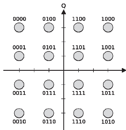
Рис. 2. Квадратурна амплітудна модуляція з 16-ти позиційним сигнальним сузір'ям
