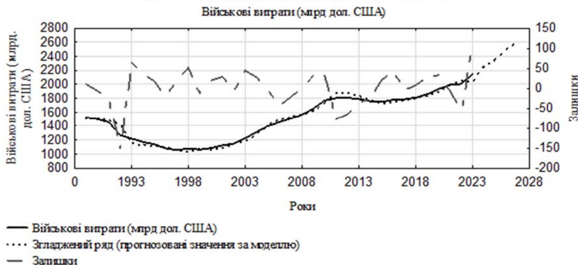
Рис. 5. Результати прогнозу світових військових витрат за експонентною моделлю 80
