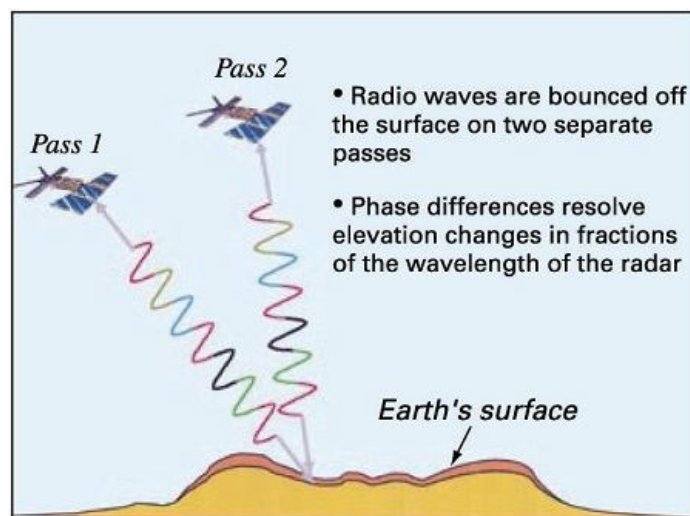
Рисунок 1 – Схематичне зображення супутника, який проходить над площею поверхні Землі (модифіковане графічне зображення [13, 14])
