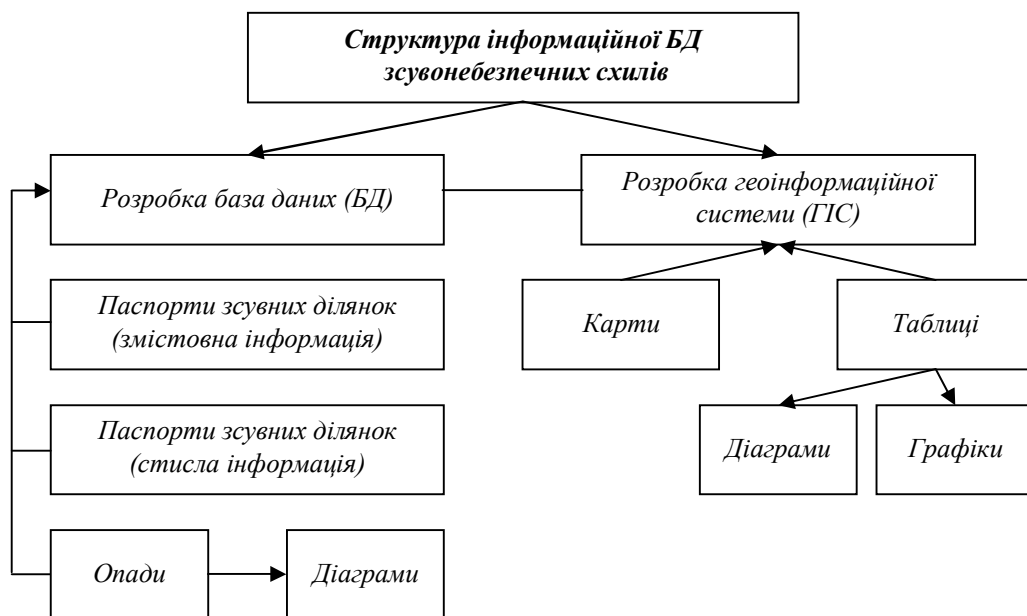
Рисунок 5 – Структура інформаційної БД зсувонебезпечних схилів
