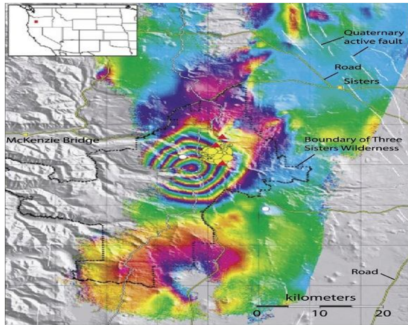
Рисунок 3 – Інтерферограма від InSAR (1997 – 2001) показує область підняття в Three Sisters вулканах (червоні трикутники), у Cascade горах, у центральному Орегоні, штат США (круги показують місця землетрусів). (Відредаговане фото з посилання [13, 14])
