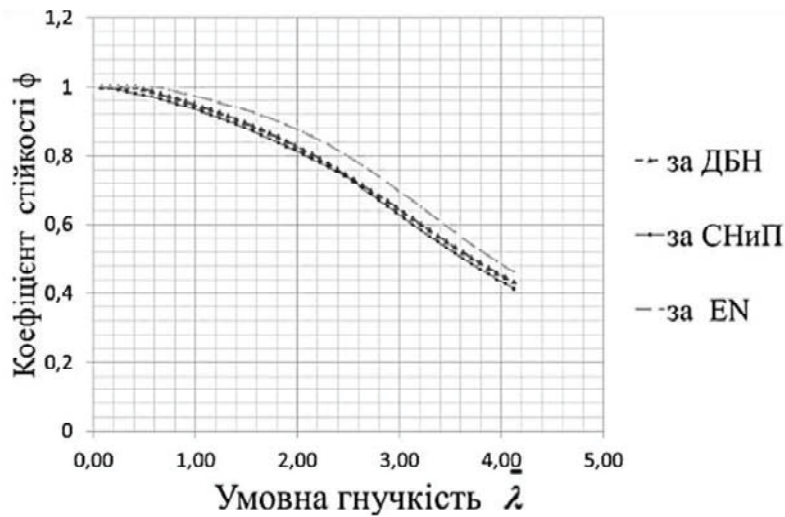
Рис. 2 – Графік залежності коефіцієнта \phi від умовної гнучкості для ЦСЕ з двотавра № 20 ГОСТ 8239-89
