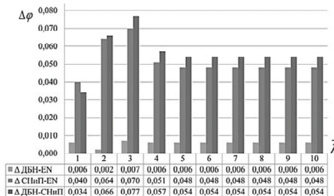
Рис. 7 – Різниця між кривими ДБН – EN, СНиП – EN і ДБН – СНиП для ЦСЕ з труби 140х6 ГОСТ 8732-78
