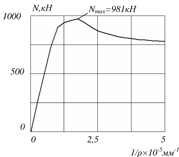
Рис. 4. Залежність поздовжньої сили від кривизни стержня
