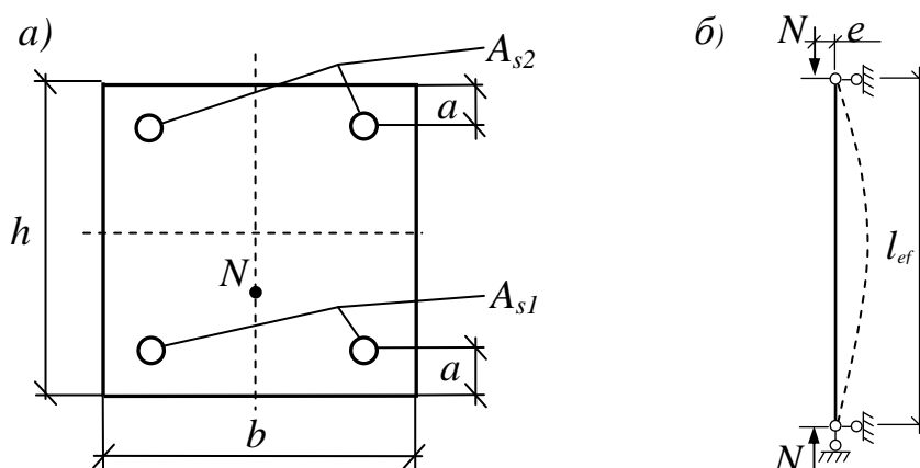
Рис. 1. Схема для розрахунку несучої здатності позацентрово стиснутих елементів: а – схема перерізу; б – розрахункова схема стержня
