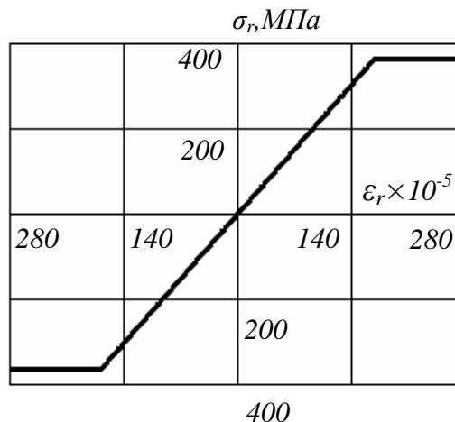
Рис. 3. Діаграма залежності \sigma_r - \epsilon_r сталевого елемента
