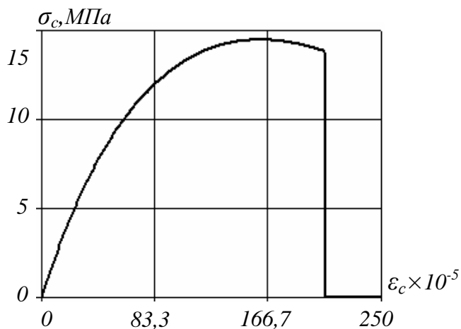
Рис. 2. Повна діаграма залежності \sigma_c - \epsilon_c стиснутого бетону
