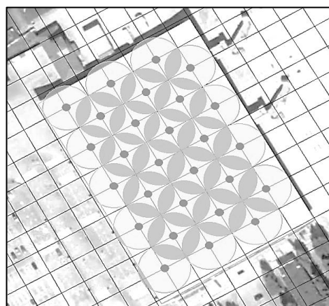
Рис. 40. Картографічна схема розташування роутерів Wi-Fi та зон їх дії в аеропорті міста Харкова ( Fig. 40. Cartographic layout of Wi-Fi routers and their areas of operation at the airport of Kharkiv)
