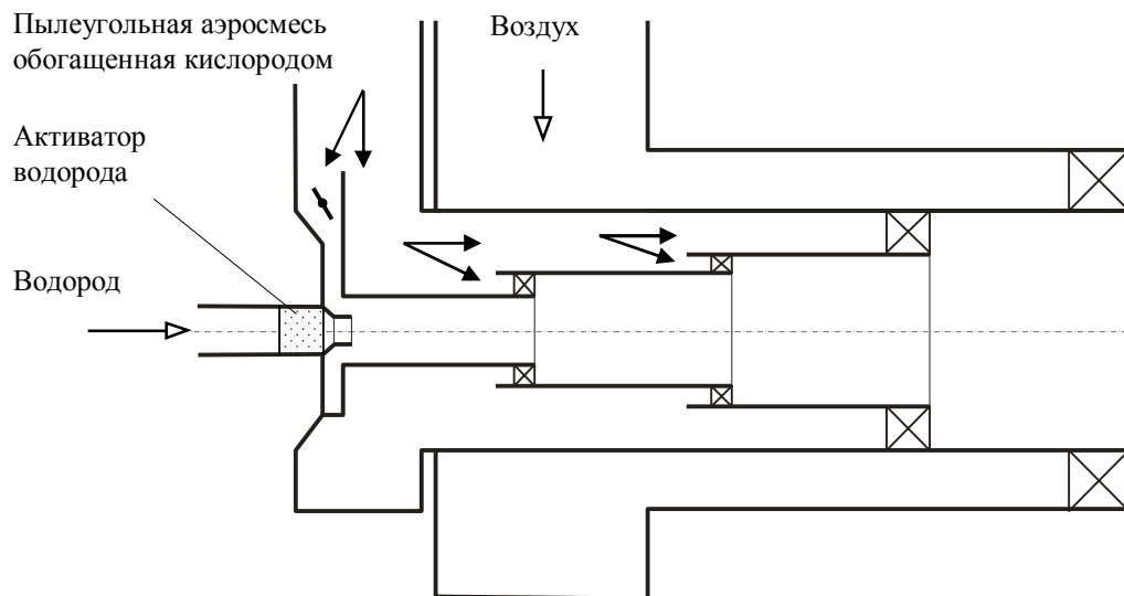
Рис. 6. Схема реактора водородно-кислородной ТХП пылеугольновоздушной смеси
