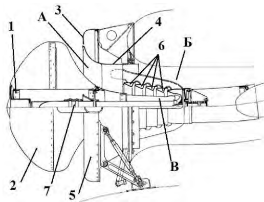
Рис. 2. Схема работы пылезащитного устройства инерционного типа:
