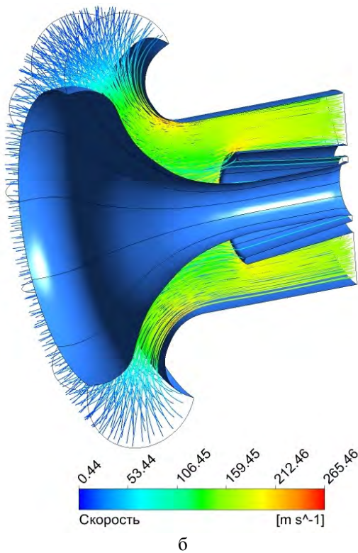
Рис. 6.Траектория и скорость движения: а –частиц во входном устройстве ГТД с ПЗУ (размер частиц 10...50 мкм); б –линий воздушного потока
