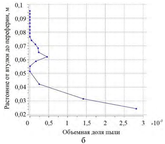
Рис.7. Распределение удельного объема частиц размером 10...50 мк: а – в продольном сечении входного устройства ГТД; б –радиальная зависимость удельного объема посторонних частиц на выходе из входного аппарата
