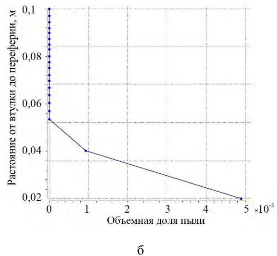
Рис. 9. Распределение удельного объема частиц размером 50...100 мк: а – в продольном сечении входного устройства ГТД; б – радиальная зависимость удельного объема посторонних частиц на выходе из входного аппарата
