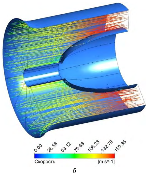
Рис. 5. Распределение скорости частиц во входном тоннеле без ПЗУ для частиц размером: а – 10...50 мкм; б – 50...100 мкм
