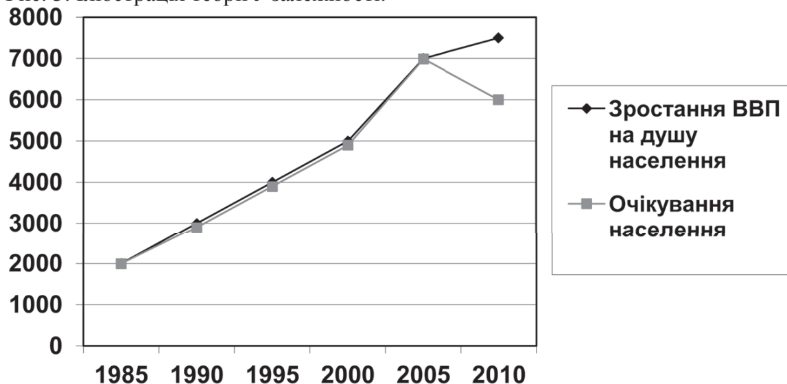
Рис. 5. Ілюстрація теорії J-залежності.
