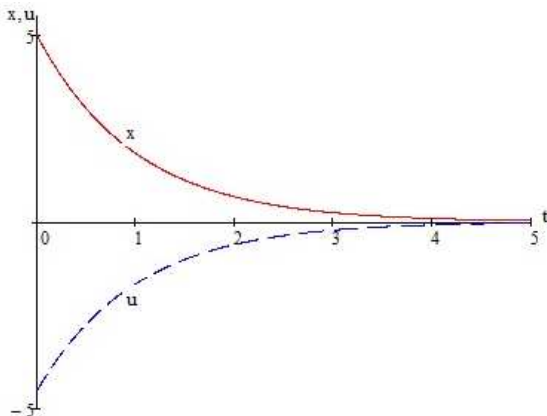
Рис. 2 – Графіки переменной состояния и управления при допустимом расходе энергии и полученном коэффициенте усиления алгоритма управления
