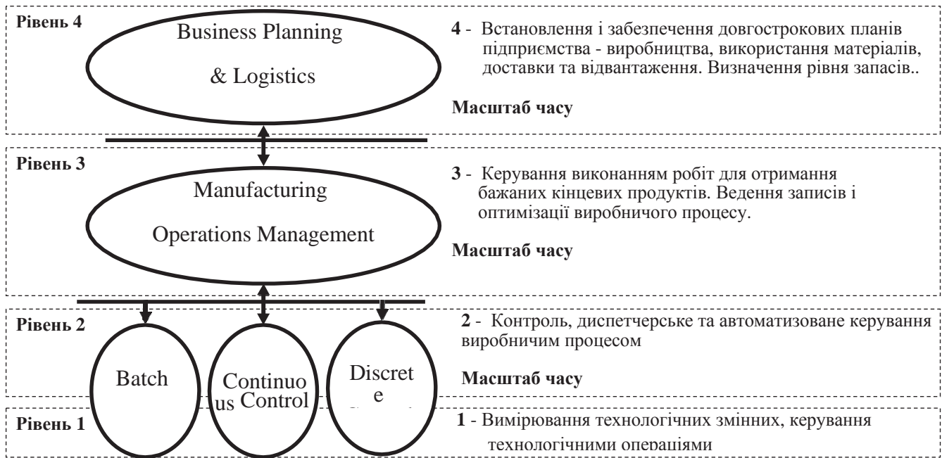
Рис.1 - Функціональна ієрархічна структура керування виробничим підприємством згідно ISA-95 (МЕК 62264)
