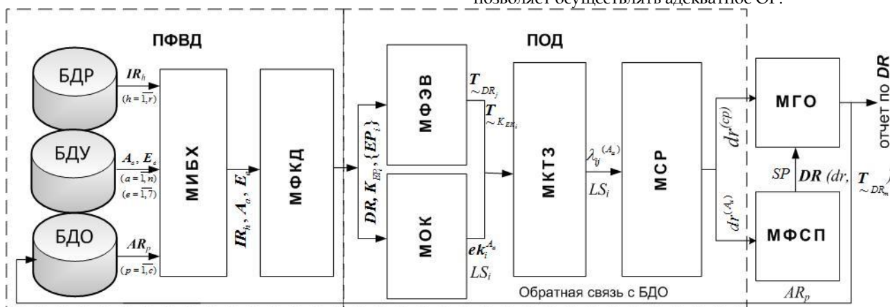
Рис. 1. Структурная схема ИАСОР
