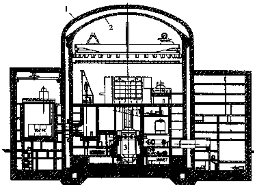
Рис. 3. Реакторное отделение энергоблока с двойной защитной оболочкой: 1 – внешняя оболочка; 2 – внутренняя оболочка
