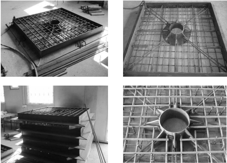
Рис. 1. Надколонні плити для безбалкового перекриття ресторану під час їх виготовлення
