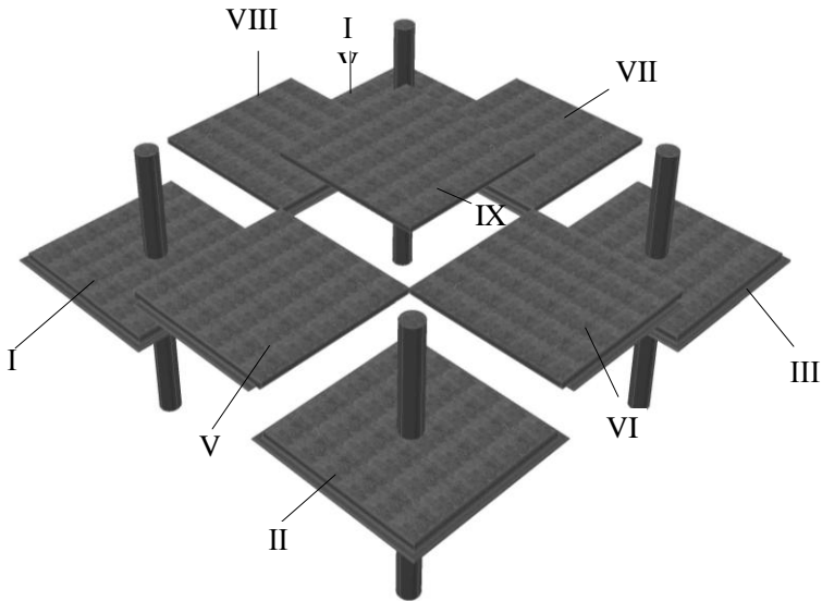
Рис. 2. Монтаж сталезалізобетонного безбалкового перекриття: I, II, III ... – черговість монтажу плит
