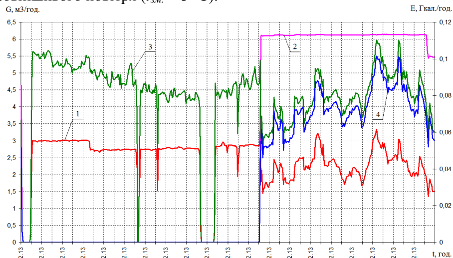
Рис. 1. Витрати теплоносія та теплоти в подавальному (до ІТП) та змішувальному зворотному (після ІТП) трубопроводах:
