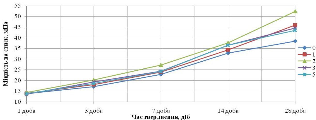
Рис. 2. Вплив кількості додатку вапна, віброактивованого 45 хвилин, на процес тверднення цементного тіста
