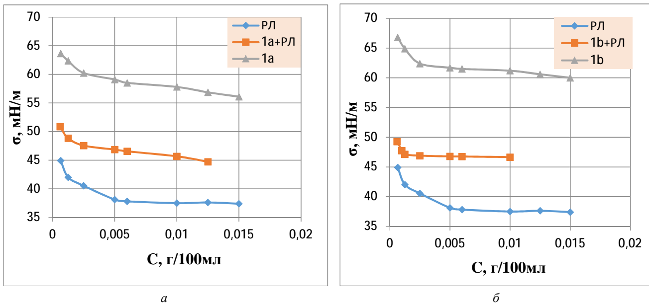
Рис. 1. Ізотерми поверхнього натягу гетероциклічних амінопохідних нафтохінону 1a, b (а), рамноліпиду РЛ та комплексних препаратів на їх основі 1a,b+РЛ (б)
