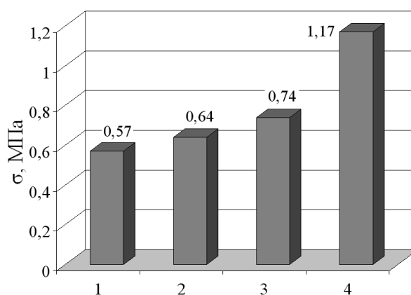
Рис. 2. Вплив молекулярної маси ПВП і товщини композиційних плівок на їх міцність під час проривання, \sigma , МПа: Гідрогель: MM_{ПВП} : 1 – 12 \cdot 10^3 , 2–4 – 3,6 \cdot 10^5 ; Розчин: MM_{ПВП} , г/моль: 1,2 – 3,6 \cdot 10^5 , 3,4 – 12 \cdot 10^3 ; \delta , мм: 1–3 – 0,5, 4 – 0,3
