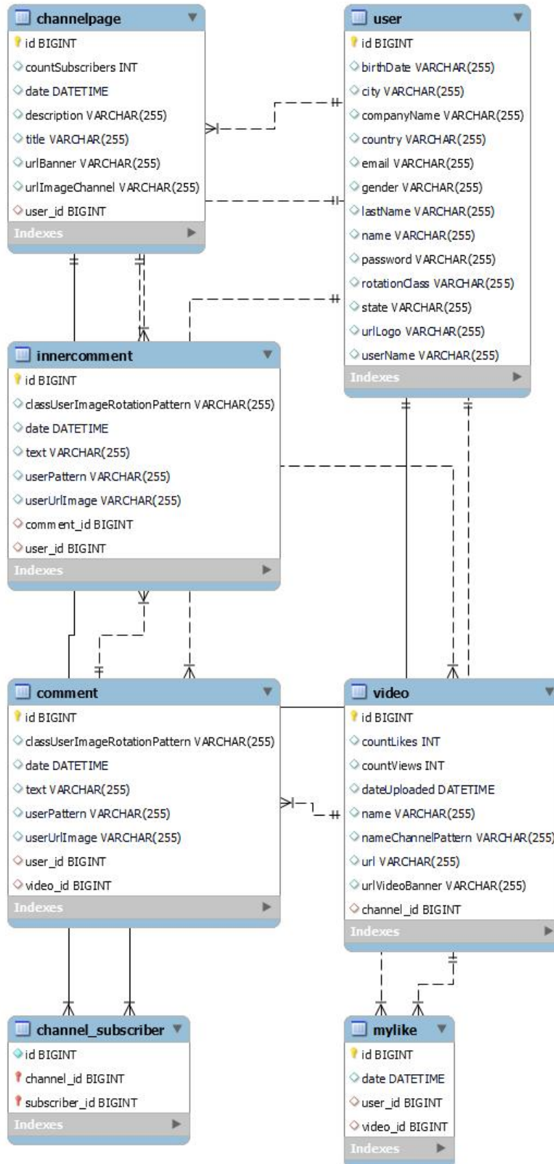
Рис. 3. Структура бази даних онлайн-платформи відеогостингу з контекстно-залежним рекомендаціям відеоданих
