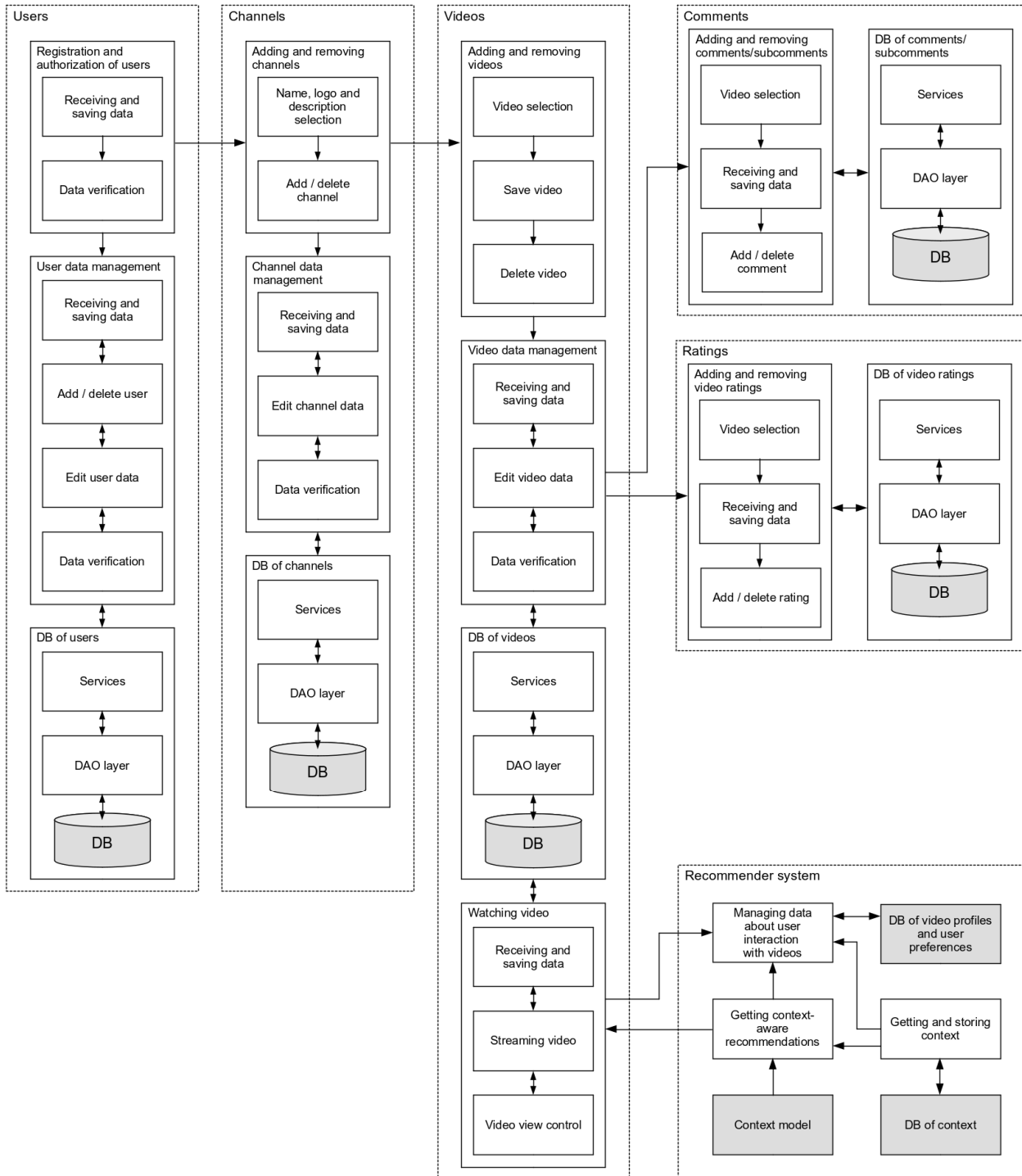
Рис. 2. Структурна схема серверної частини онлайн-платформи відеогостингу з контекстно-залежним рекомендуванням відеоданих
