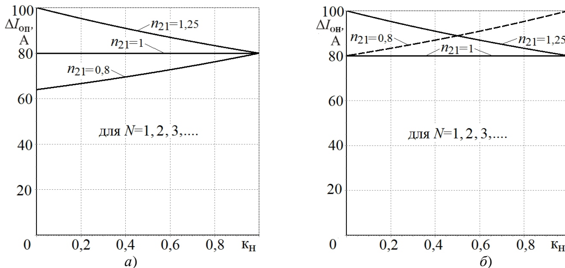
Рисунок 5 – Зависимости пульсаций токов потребления \Delta I_{\text{он}} (а) и нагрузки \Delta I_{\text{он}} (б) ППН модульной структуры при однофазном принципе преобразования при P_{\text{н}} = \text{const} = 400\text{ Вт}
