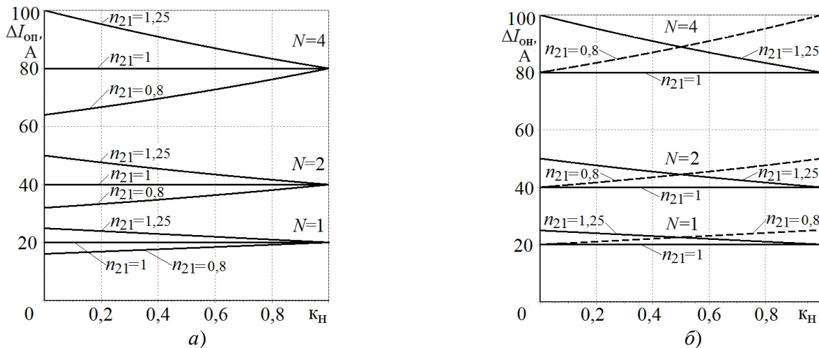
Рисунок 4 – Зависимости пульсаций токов потребления \Delta I_{оп} (а) и нагрузки \Delta I_{он} (б) ОИП при P_{пк}=100 Вт
