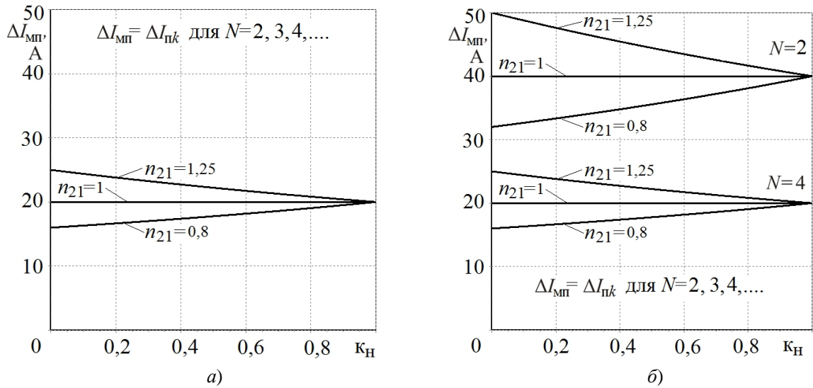
Рисунок 8 – Зависимости пульсаций токов потребления \Delta I_{мп} многофазного импульсного преобразователя при P_{нк}=100 Вт (а) и P_n=400 Вт (б)
