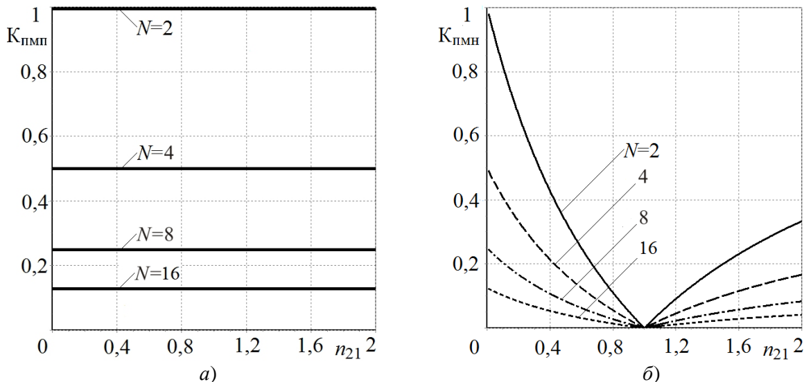
Рисунок 14 – Зависимости коэффициентов пульсаций токов на входе K_{\text{пмп}} (а) и выходе K_{\text{пмп}} (б) ППН модульной структуры – МИП от коэффициента трансформации n_{21} при k_{\text{п}} = 0,5
