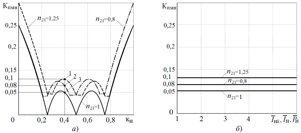
Рисунок 12 – Зависимости коэффициентов пульсаций токов на выходе K_{\text{пмн}} от коэффициента накопления – K_{\text{н}} (а) и относительных \bar{I}_{\text{нк}}, \bar{I}_{\text{н}}, \bar{P}_{\text{н}} МИП при N = 4
