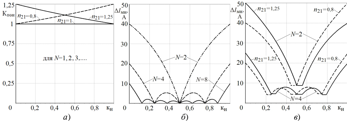
Рисунок 10 – Зависимости пульсаций токов нагрузки \Delta I_{мн} МИП при P_n = \text{const} = 800 Вт (при n_{21} = 1 (б) и n_{21} = 1,25; 0,8 (в)) в ОИП (а) и МИП (б, в)
