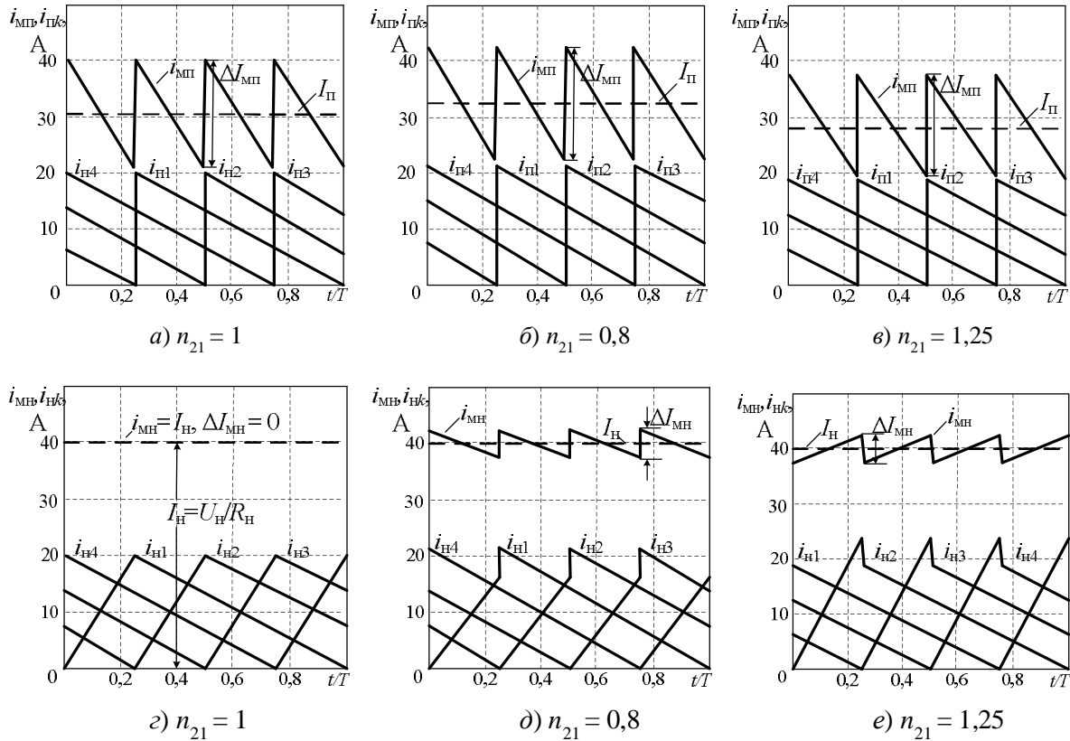
Рисунок 7 – Временные диаграммы токов МИП во входных i_{\text{мп}}(t) (а, б, в) и в выходных i_{\text{мн}}(t) (з, д, е) цепях при N = 4 , U_{\text{н}} = \text{const} , \kappa_{\text{нк}} = 0,25
