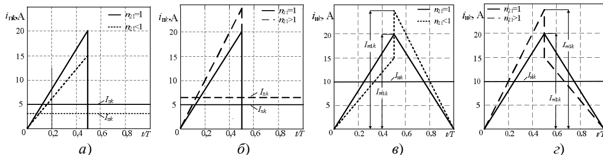
Рисунок 6 – Временные диаграммы токов потребления i_{\text{нк}}(t) (а, б) и нагрузки i_{\text{нк}}(t) (в, г) в k -х силовых каналах при различных коэффициентах трансформации n_{21}
