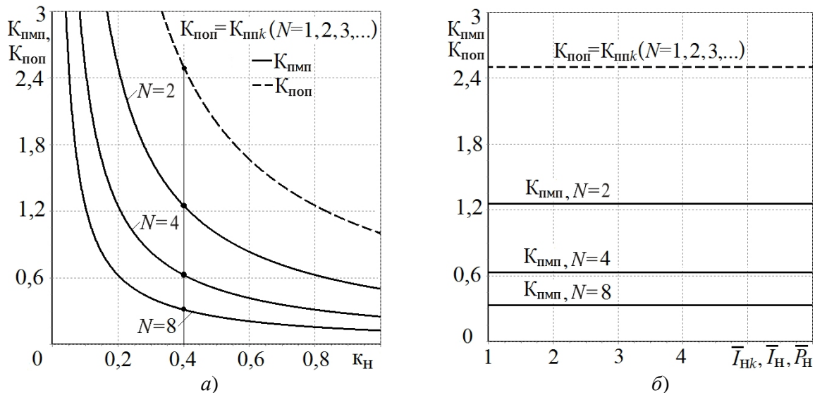
Рисунок 11 – Зависимости коэффициентов пульсаций токов на входе K_{\text{пмп}} МИП,
