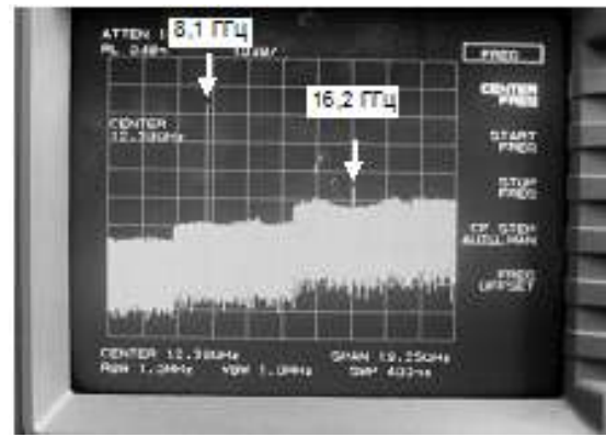
Рисунок 10 – Спектр сигналу гетеродина в області частоти 8,1 ГГц (розмах спектра на екрані 19 ГГц)
