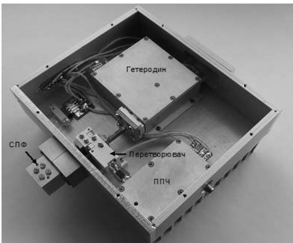
Рисунок 17 – Розташування вузлів у складі приймального (передавального) трактів
