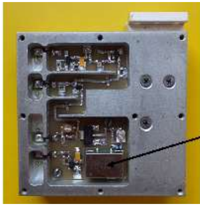
Рисунок 9 – Задавальний генератор, змонтований на зворотній стороні корпусу гетеродина
