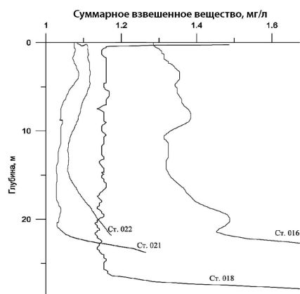
Р и с . 4 . Вертикальные профили взвешенного вещества.
