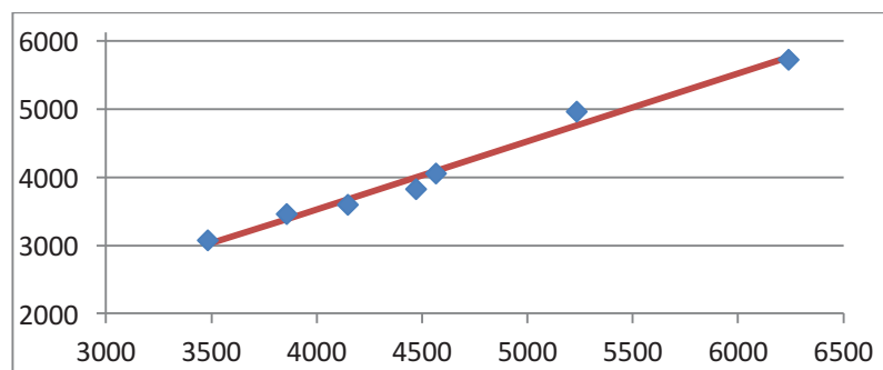
Рис.1 Лінія регресії
