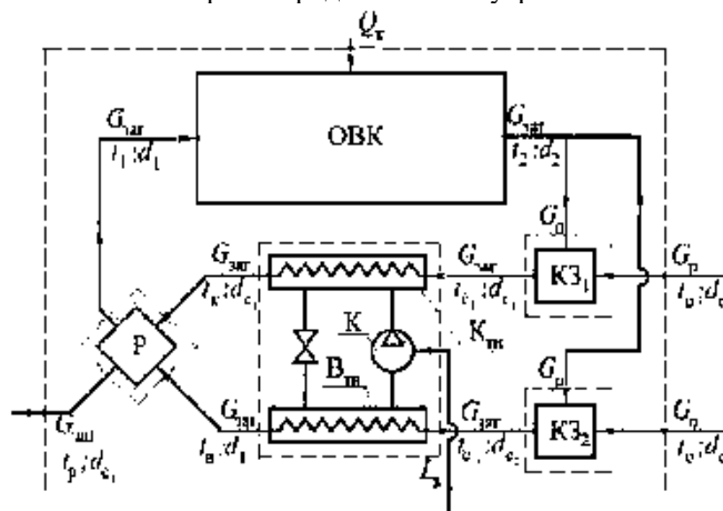
Рис. 1. Принципова ТНУ вентиляції та кондиціонування повітря в приміщенні: K_{тн} – конденсатор ТН; B_{тн} – випарник ТН; K – компресор; KЗ_1 – перша камера змішування; KЗ_2 – друга камера змішування; P – рекуператор; OBK – об’єкт вентиляції та кондиціонування повітря
