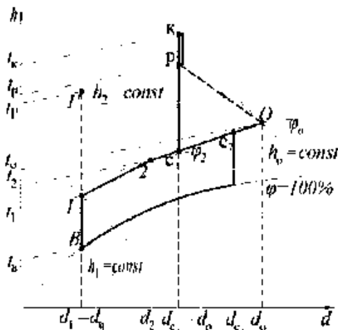
Рис. 2. Робочий процес зміни стану повітря в системі вентиляції та кондиціонування приміщення в h-d діаграмі
