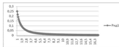
Рис. 4. Щільність розподілу Паретто
