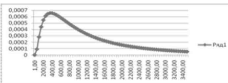
Рис. 3. Щільність Лог-нормального розподілу
