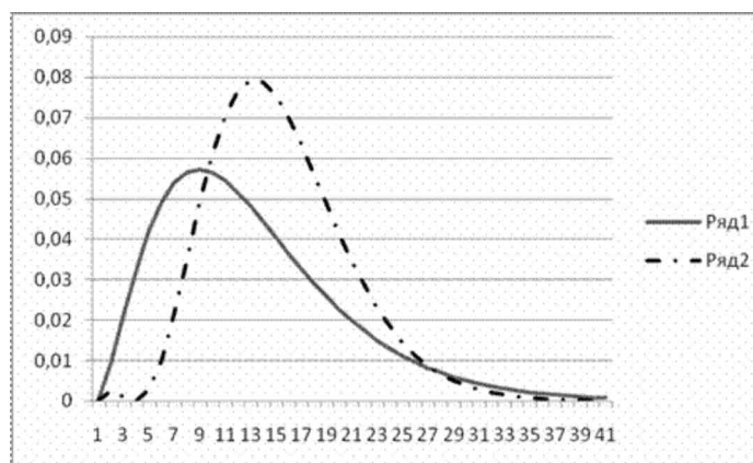
Рис. 10. Співвідношення двох щільностей функцій розподілу
