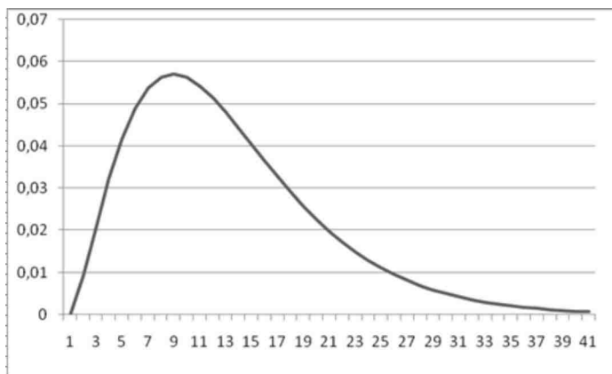
Рис. 9 Графік апроксимованої функції розподілу
