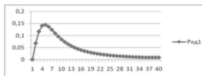
Рис. 7. Щільність розподілу Бурра
