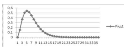
Рис. 8. Графік функції розподілу
