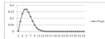
Рис. 6. Щільність розподілу Вейбула
