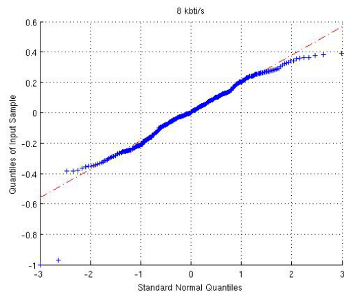
Рис. 13. Квантили розподілення нормального закону і отриманих даних 8 кбіт/с
