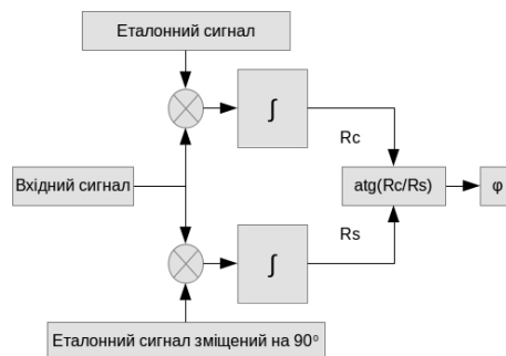
Рис 1. Схема роботи синхронно-квадратурного детектора
