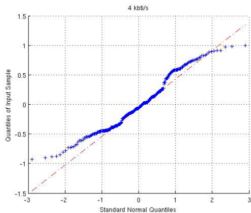
Рис. 12. Квантили розподілення нормального закону і отриманих даних 4 кбіт/с
