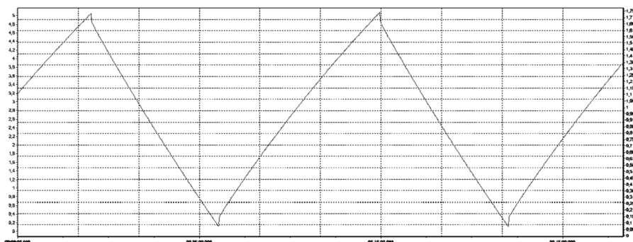
Рис. 6. Осцилограма напруги дослідного СК у зарядно-розрядних циклах зі струмом 1А
