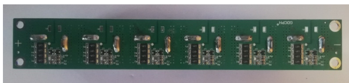
Рис. 11. Перший СК-модуль із шести послідовно з'єднаних СК (а), встановлених на платі захисту і балансування (б)
