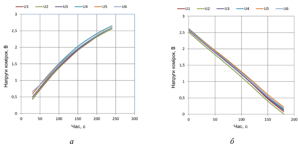
Рис. 15. Напруги на шести послідовно з'єднаних СК-групах, отримані експериментально під час заряджання (а) і розряджання (б) другого СК-модуля струмом 3,3 А
