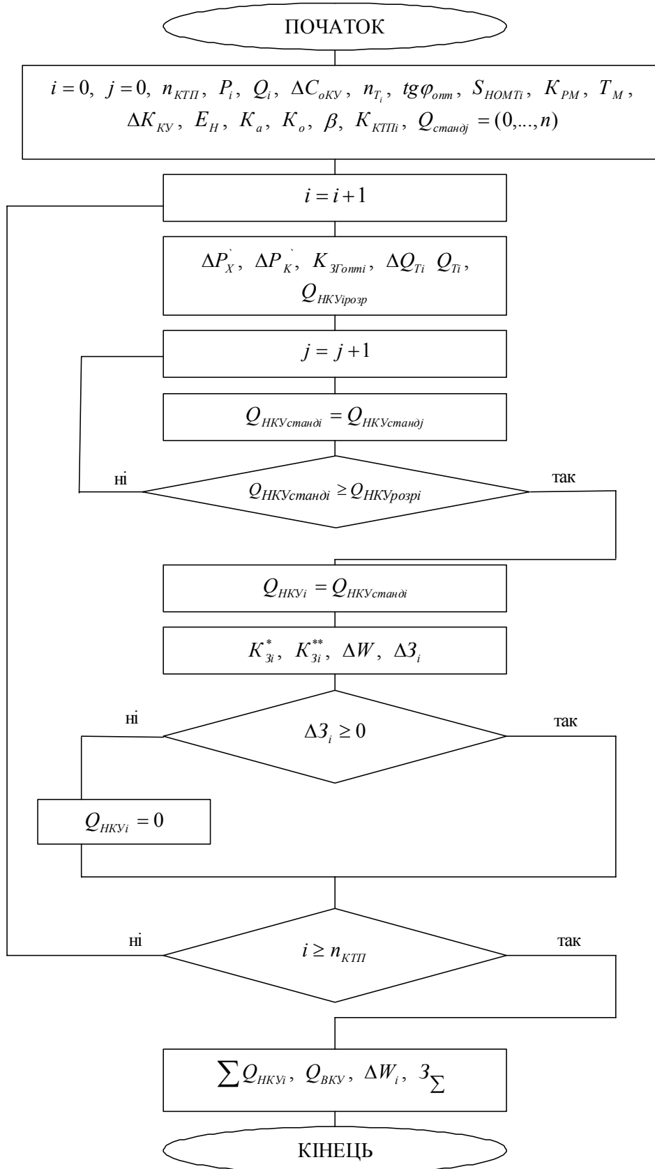
Рис. 1. Алгоритм вибору компенсуючих пристроїв: де K_{рм} – коефіцієнт різночасності максимумів навантаження; tg\varphi_{опт} – оптимальний коефіцієнт реактивної потужності, який задається енергопостачальною організацією; n_{КТП} – кількість КТП
