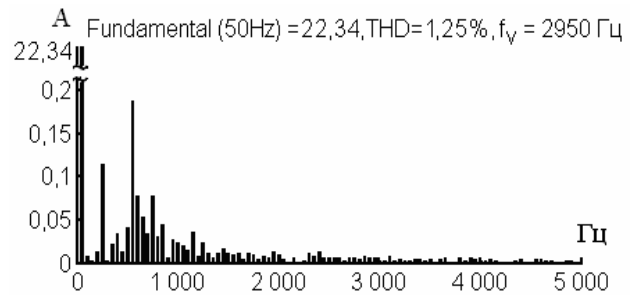
Рис.3. Спектрограмма СФТ при питании частотно-регулируемого асинхронного АЭП
