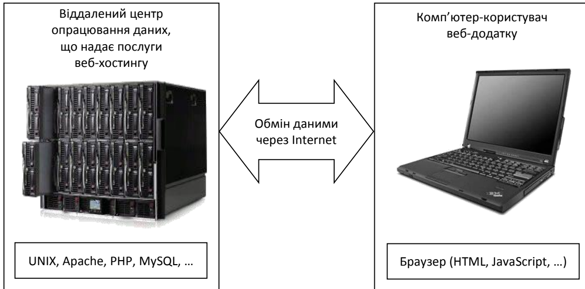
Рис. 1. Функціонування web-сторінки
