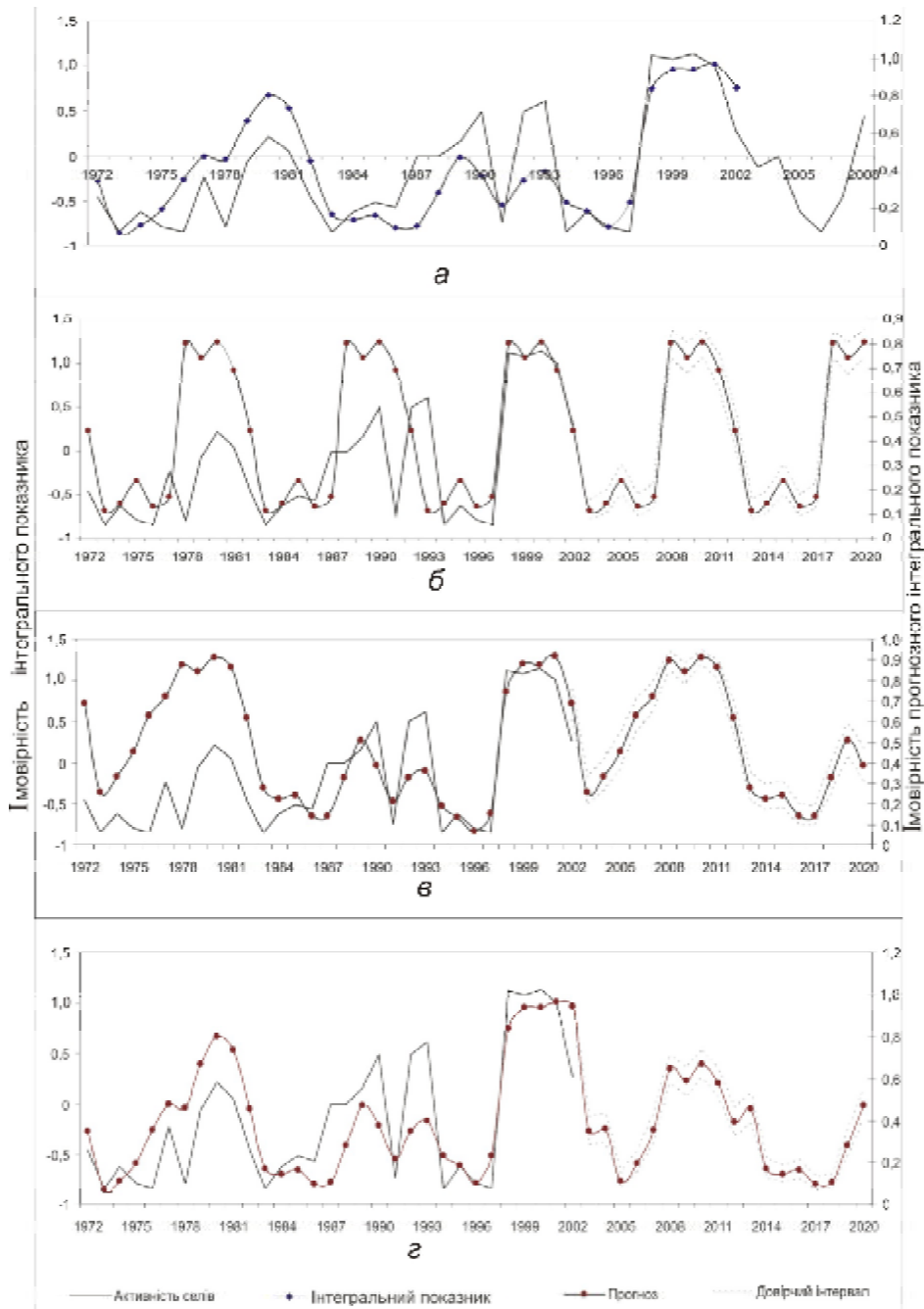
Рис. 9. Часові ряди: активності селів та інтегрального показника: а – 1972–2008 рр.; б–г – прогнози (б – осередненням ряду, в – аналізом Фур'є, г – багаточаровим перцептроном)
