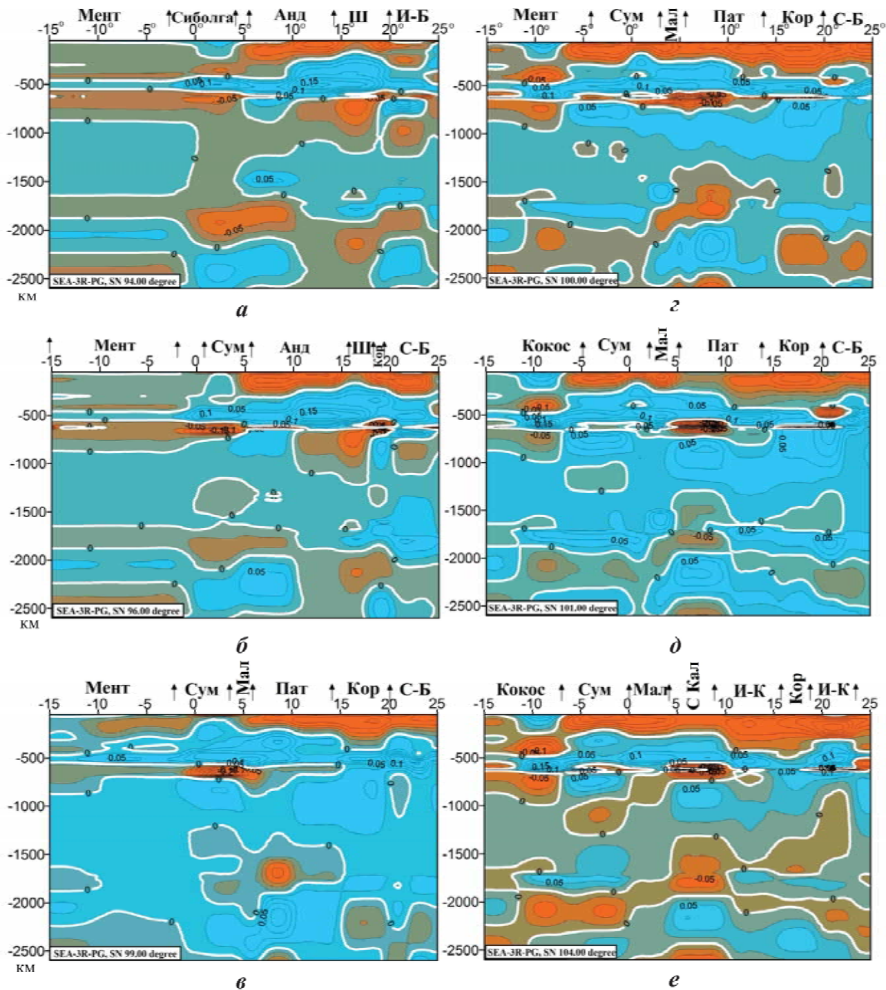
Рис. 2. Долготные сечения 94° (а), 96° (б), 99° (в), 100° (г), 101° (д), 104° (е) трехмерной модели мантии Юго-Восточной Азии. Блоки: Анд – Андаман, И-Б – Индо-Бирманья; И-К – Индокитай, Кор – Корат, Мал – Малайзия, Мент – Ментавай, Пат – Паттани, С-Б – Синобирманья, С Кал – Северный Калимантан, Сум – Суматра, Ш – Шан Тхай Fig. 2. Longitudinal cross section 94° (a), 96° (b), 99° (v), 100° (z), 101° (d), 104° (e) three-dimensional model of the mantle Southeast Asia. Blocks: And – Andaman, I-B – Indobirmaniya, I-C – Indochina, Kor – Korat, Mal – Malaysia, Ment – Mentawai, Pat – Pattani, S-B – Sinobirmaniya, N Kal – North Kalimantan, Sum – Sumatra, Sh – Shan Thai
