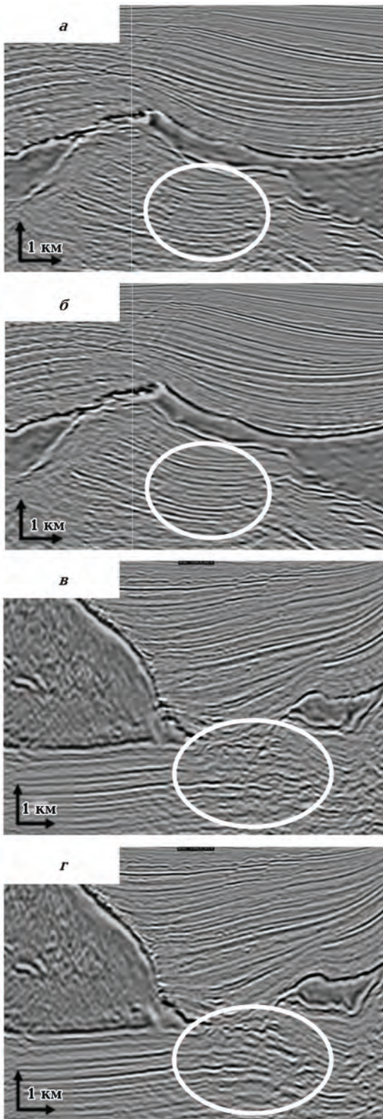
Рис. 14. Результаты миграции в обратном времени в Мексиканском заливе в направлении инлайн со скоростными моделями ТПИ (а) и T-ORT (б) и в направлении кросслайн со скоростными моделями ТПИ (в) и T-ORT (г). Соль обозначена более темным цветом.
