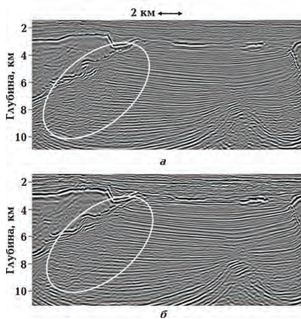
Рис. 10. Сейсмические изображения, полученные в Мексиканском заливе после применения миграции в обратном времени с VTI ( a ) и TPI ( б ) моделью скоростной анизотропии.
