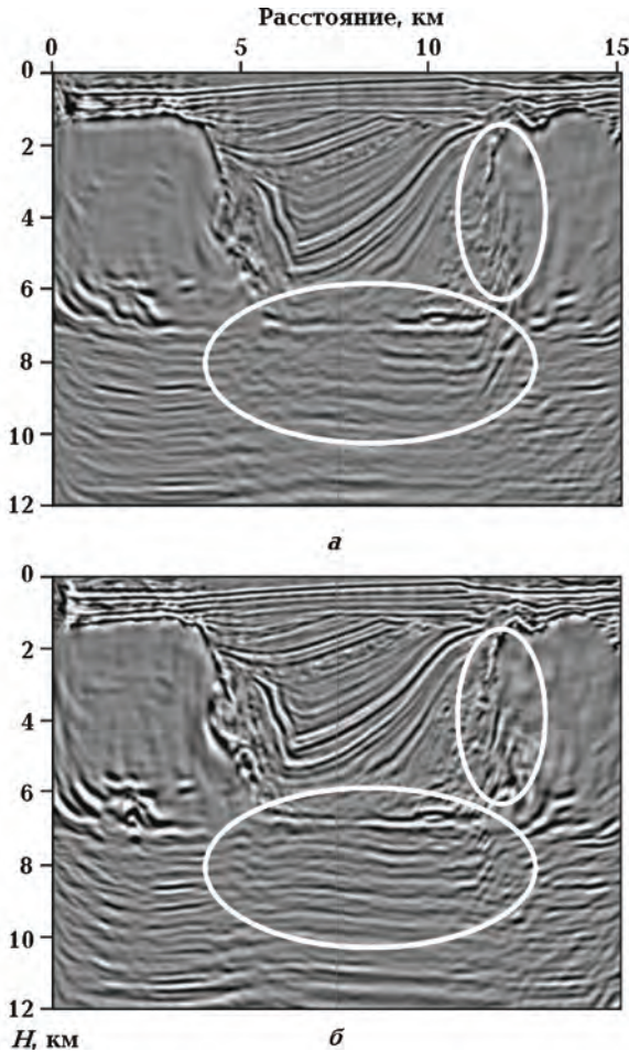
Рис. 11. Сейсмические изображения, полученные в Мексиканском заливе после применения миграции в обратном времени с VTI (а) и HTI (б) моделью скоростной анизотропии.
