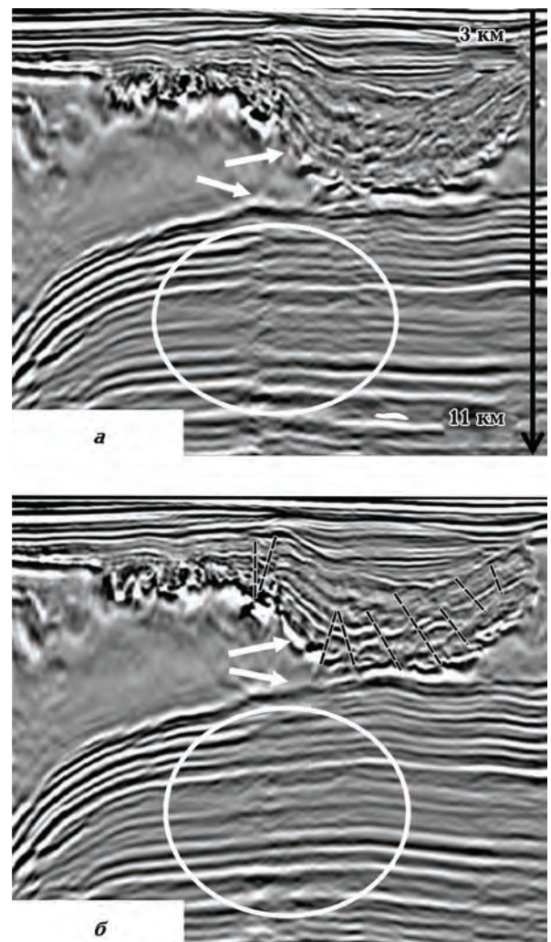
Рис. 15. Сейсмические изображения, полученные со скоростными моделями ТПИ (а) и T-ORT (б) в Мексиканском заливе. Черными пунктирными линиями обозначены тектонические нарушения, а стрелками и эллипсом — места улучшения изображения после миграции с T-ORT скоростной моделью.
