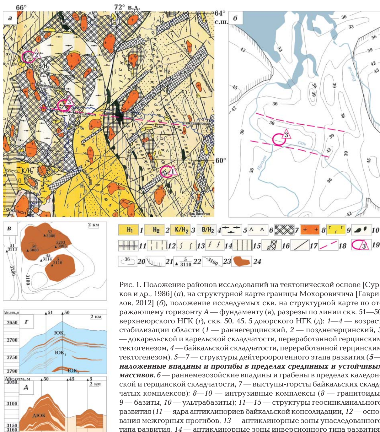
Рис. 1. Положение районов исследований на тектонической основе [Сурков и др., 1986] (а), на структурной карте границы Мохоровичича [Гаврилов, 2012] (б), положение исследуемых скв. на структурной карте по отражающему горизонту А — фундаменту (в), разрезы по линии скв. 51—50 верхнеюрского НГК (r), скв. 50, 45, 5 доюрского НГК (Δ): 1—4 — возраст стабилизации области (1 — раннегерцинский, 2 — позднегерцинский, 3 — докарельской и карельской складчатости, переработанной герцинским тектогенезом, 4 — байкальской складчатости, переработанной герцинским тектогенезом). 5—7 — структуры дейтероорогенного этапа развития (5 — наложенные впадины и прогибы в пределах срединных и устойчивых массивов , 6 — раннемезозойские впадины и грабены в пределах каледонской и герцинской складчатости, 7 — выступы-горсты байкальских складчатых комплексов); 8—10 — интрузивные комплексы (8 — гранитоиды, 9 — базиты, 10 — ультрабазиты); 11—15 — структуры геосинклинального развития (11 — ядра антиклинорий байкальской консолидации, 12 — основания межгорных прогибов, 13 — антиклинорные зоны унаследованного типа развития, 14 — антиклинорные зоны инверсионного типа развития, 15 — синклинорные зоны унаследованного типа развития); 16 — раннемезозойские грабен-рифты ; 17 — дизъюнктивная тектоника; 18 — граница сутурной зоны [Гаврилов, 2012]; 19 — район исследований: Чистинная группа месторождений [Коржов и др., 2019] (1), Рогожниковская группа месторождений [Коржов и др., 2013] (2), Ханты-Мансийское месторождение (3); 20 — изогипсы на поверхности Мохоровичича, км; 21 — обрамление ЗСП; 22 — исследуемая скважина (в числителе — номер, в знаменателе — отметка кровли доюрского фундамента); 23 — изогипсы кровли доюрских отложений, м; 24 — залежь нефти.
