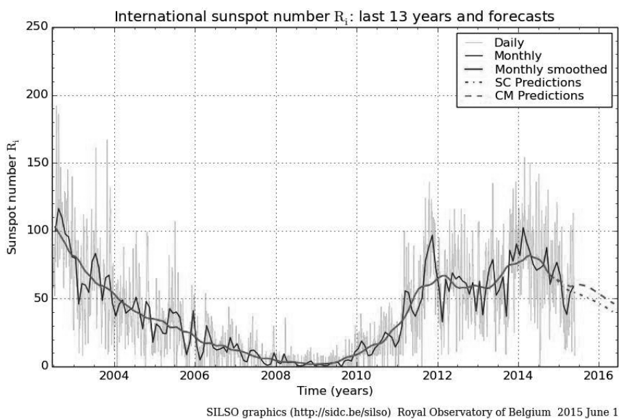
Рис. 2. Дані спостереження за Сонцем від Royal Observations (Бельгія), роки/місяці [14]
