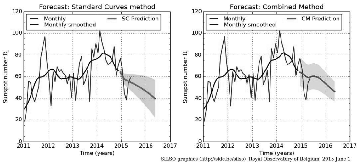
Рис. 1. Дані спостереження за Сонцем від Royal Observations (Бельгія), роки/місяці [12]
