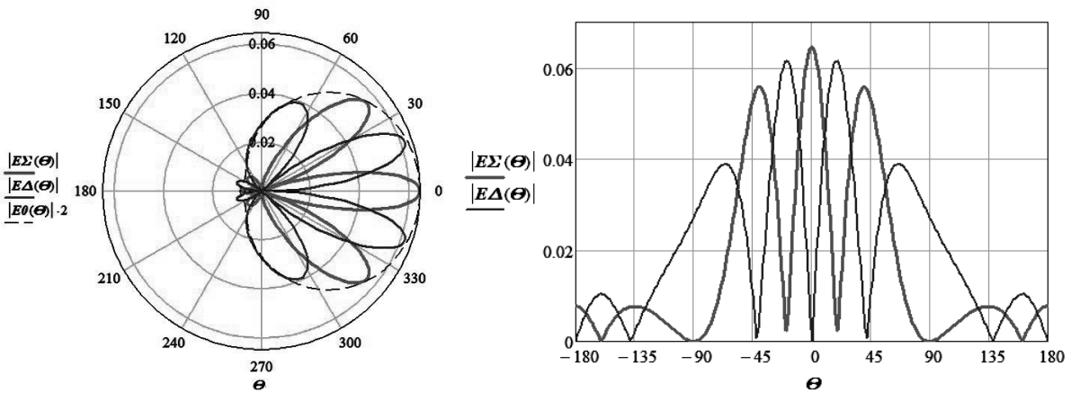
Рис. 15. Діаграми за відстані між антенами 1,5\lambda
