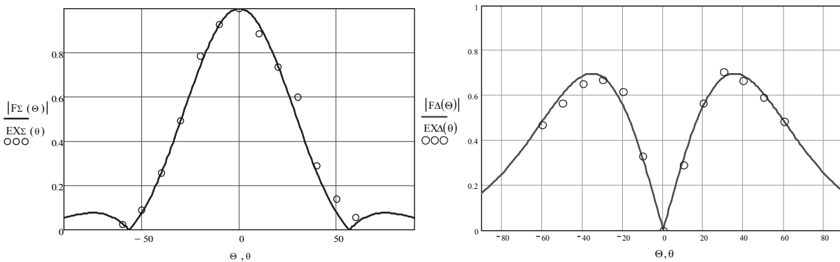
Рис. 11. Результати тестування макета з п. 4, сумарний канал
