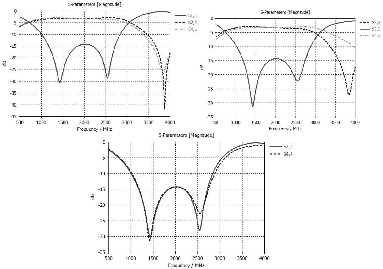
Рис. 6. S-параметри розробленого кільцевого моста, розраховані в середовищі CST Studio
