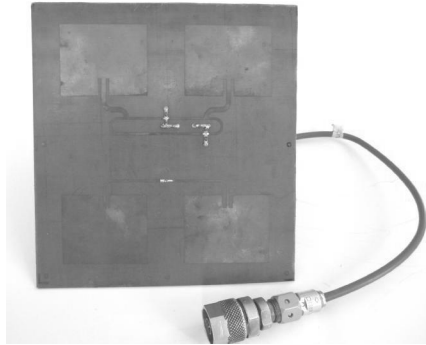
Рис. 4. Макет антенної системи радіопеленгатора за фазовим методом
