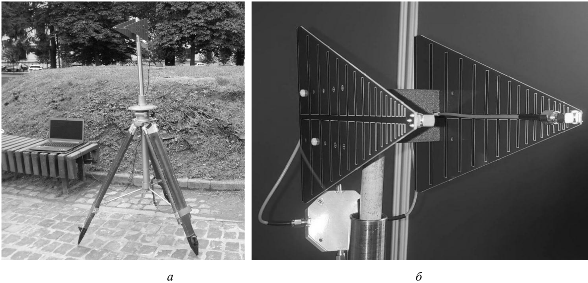
Рис. 12. Загальний вигляд стенда для тестування (а) та антенної системи з кільцевим мостом (б)
