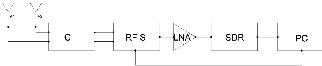
Рис. 1. Структурна схема пеленгатора
