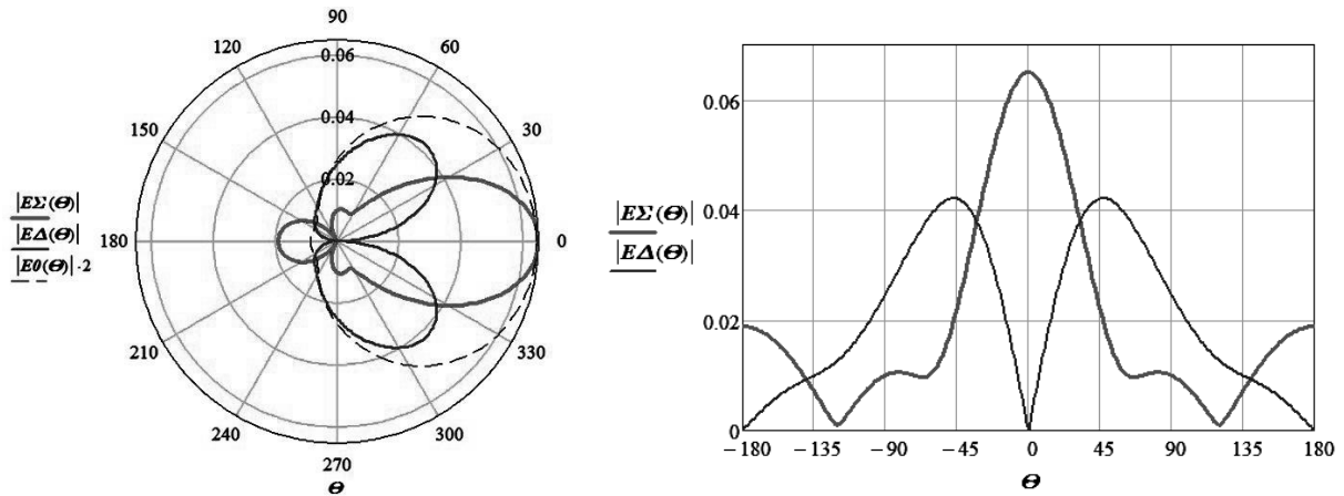
Рис. 16. Результуюча діаграма спрямованості
