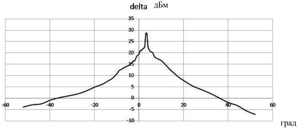
Рис. 14. Остаточний результат вимірювань
