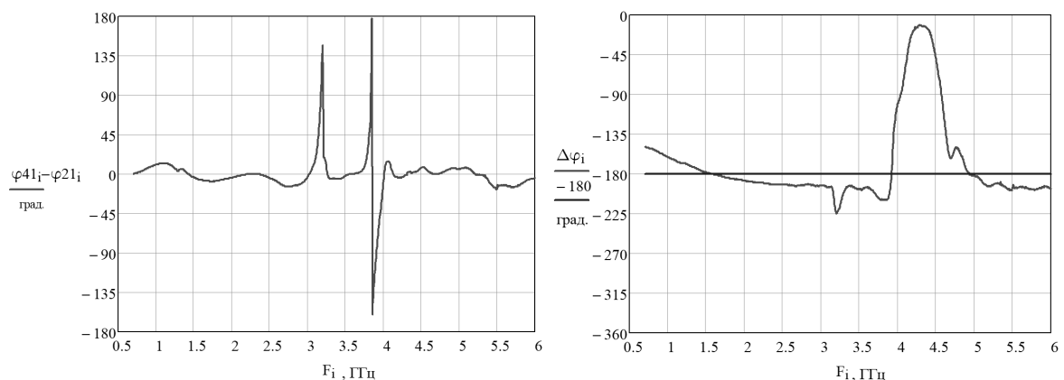
Рис. 9. ФЧХ на сумарному та різницевому каналах
