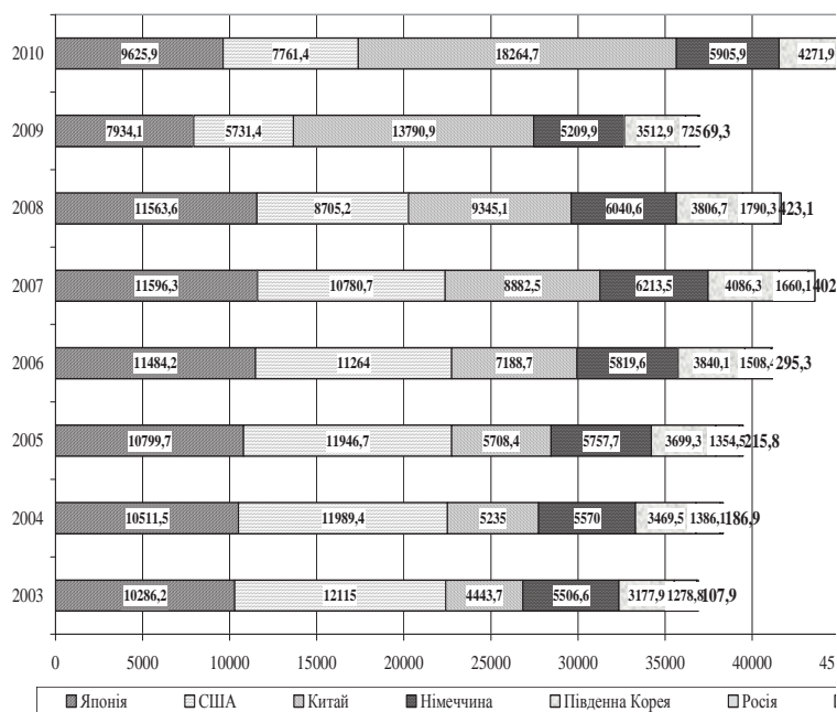
Рис. 1. Динаміка виробництва автомобілів в окремих країнах, тис. од. [1]
