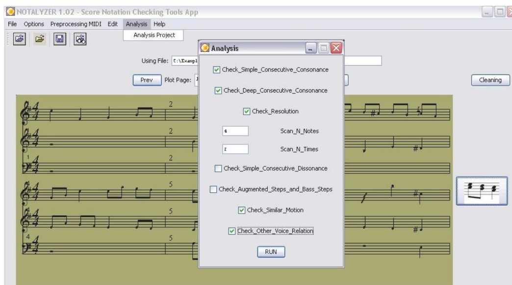
Рис. 2. Окно процедуры анализа проекта.
