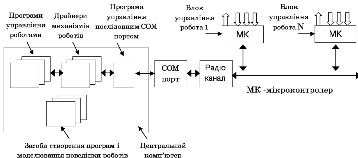
Рис. 2. Структура розподіленого централізованого управління макетами роботів
