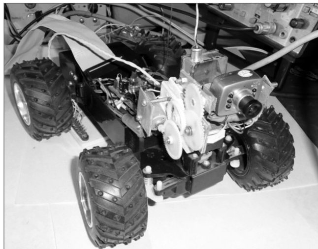
Рис. 4. Модель самохідного керованого шасі робота з відеосистемою і засобами керування камерою і передатчиком радіоканалу
