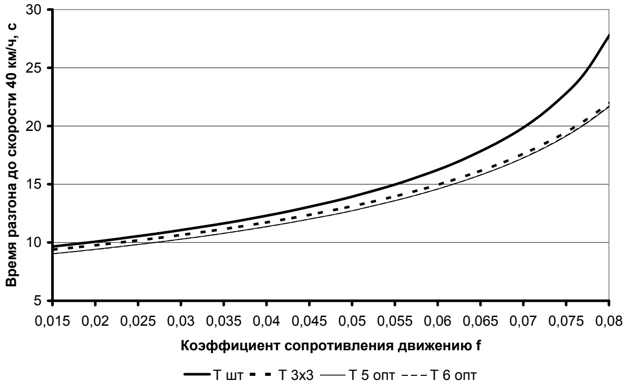
Рис. 4. Зависимости от коэффициента сопротивления движению времени достижения скорости 40 км/ч
