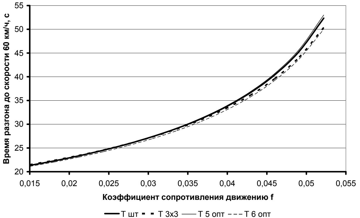
Рис. 5. Зависимости от коэффициента сопротивления движению времени достижения скорости 60 км/ч
