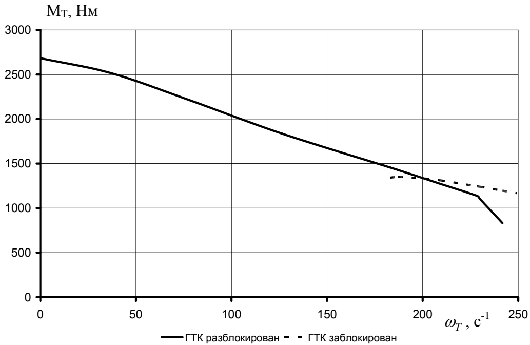
Рис. 2. Внешняя характеристика двигателя 3ТД-3 с комплексной гидродинамической передачей ГТК – XV от БМП-3
