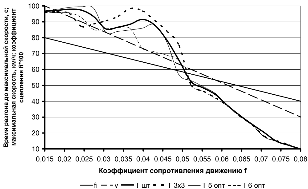
Рис. 3. Зависимости от коэффициента сопротивления движению максимально достижимой скорости, времени ее достижения и коэффициента сцепления колес с опорной поверхностью
