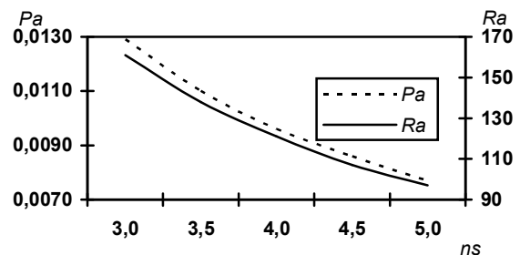
Рисунок 1 – Залежність питомої поляризованості і поляризаційного опору P_a = P_a і R_a = P_a/S_a від відношення ns , яке відповідає зростанню швидкості корозії під дією сірководню ( [P_a] = 1 \text{ Ом} \cdot \text{м}^2 ; [R_a] = 1 \text{ МОм} )
