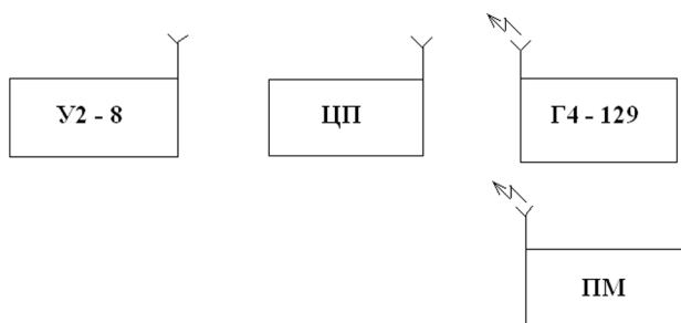
Рис. 1. Схема испытаний на помехоустойчивость экспериментальной модели АСПСР
