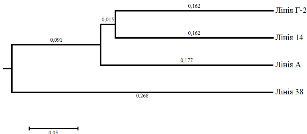
Рис. 3. Дендрограма міжпопуляційних взаємин, побудована на основі аналізу генетичних дистанцій за N_e методом незваженої попарно-групової кластеризації (UPGMA)
