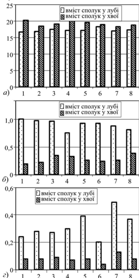
Рис. 2. Особливості накопичення водорозчинних білків і сполук фенольної природи у лубі та хво́ї сосни звичайної в осередках "короїдного" усихання: а) – вміст білків (Б), мг/г; б) – вміст проантоціанідинів (Па), мг/г; в) – вміст катехинів (Ка), мг/г; 1-8 – № дерев
