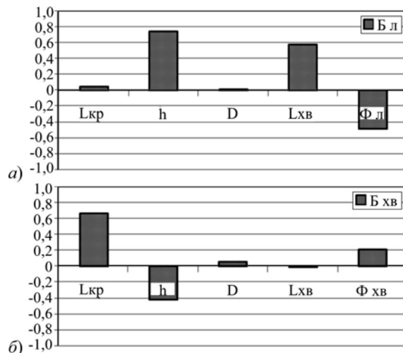
Рис. 3. Особливості кореляцій вмісту білків у лубі та хво́ї з таксаційними характеристиками дерев сосни звичайної, довжиною хво́ї та вмістом сполук фенольної природи: а) – вміст білків у лубі (Бл), мг/г; б) – вміст білків у хво́ї (Бхв), мг/г; L_{кр} – протяжність крони, м; h – висота дерев, м; D – діаметр дерев, мм; L_{хв} – довжина хво́ї мм; \Phi_l – сумарний вміст сполук фенольної природи у лубі; \Phi_{хв} – сумарний вміст сполук фенольної природи у хво́ї
