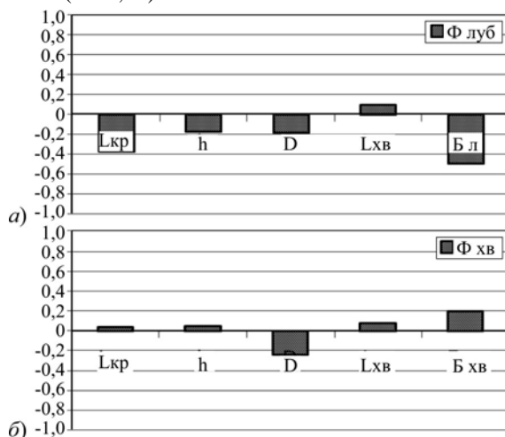
Рис. 4. Особливості кореляцій сумарного вмісту фенольних сполук у лубі та хво́ї з таксаційними характеристиками сосни звичайної, довжиною хво́ї та вмістом білків: L_{кр} – протяжність крони, м; h – висота дерев, м; D – діаметр дерев, мм; L_{хв} – довжина хво́ї мм; B_l – вміст білків у лубі; B_{хв} – вміст білків у хво́ї
