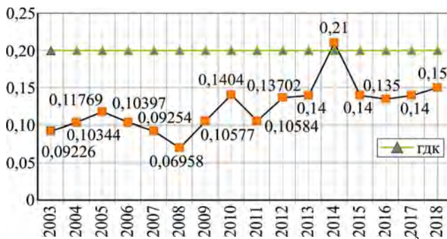
Рис. 2. Динаміка середньорічної концентрації заліза, мг/дм³
