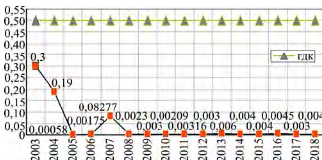
Рис. 3. Динаміка середньорічної концентрації нітритів, мг/дм³
