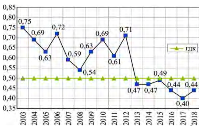
Рис. 4. Динаміка середньорічного залишкового хлору, мг/дм³
