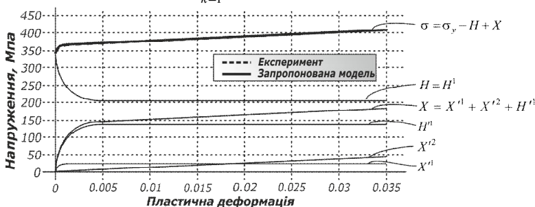
Рис. 2. Діаграма деформування
